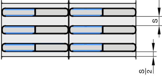
MK100: Resonantieplaten tegenover elkaar liggend
